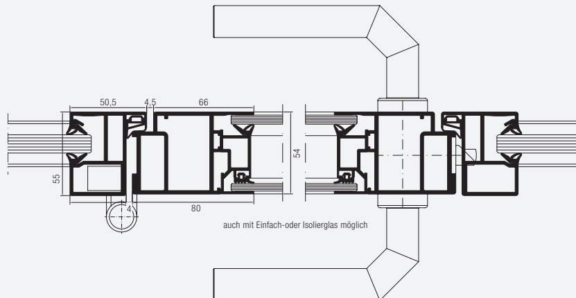
Horizontalschnitt einflügelig
