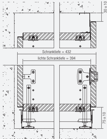
Vertikalschnitt Vorwandschrank
