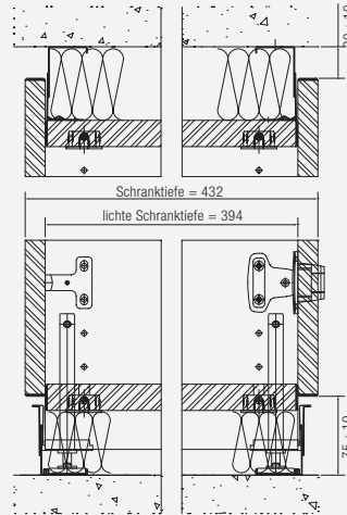
Vertikalschnitt Raumteiler
